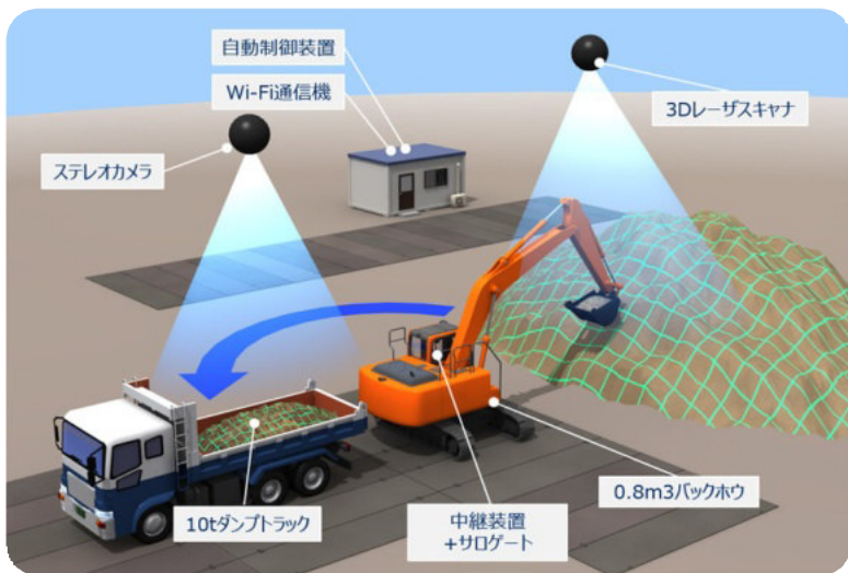
大林組、NECが共同開発した自動土砂積込システム
